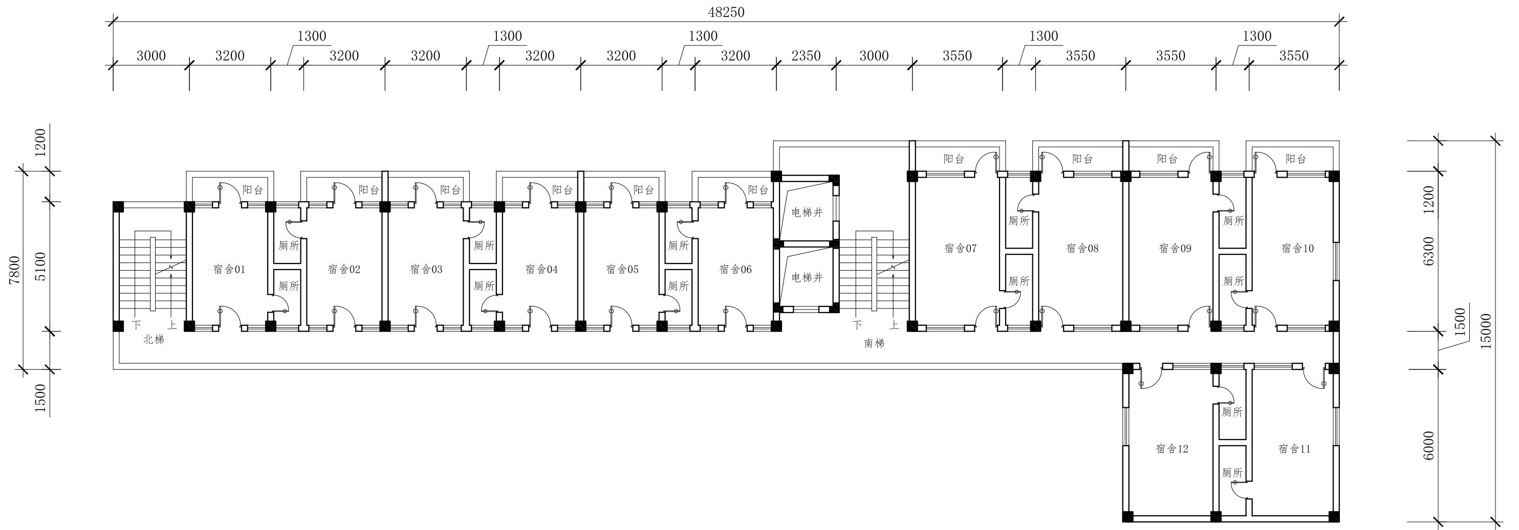
附中男生宿舍一 - 九层平面图
