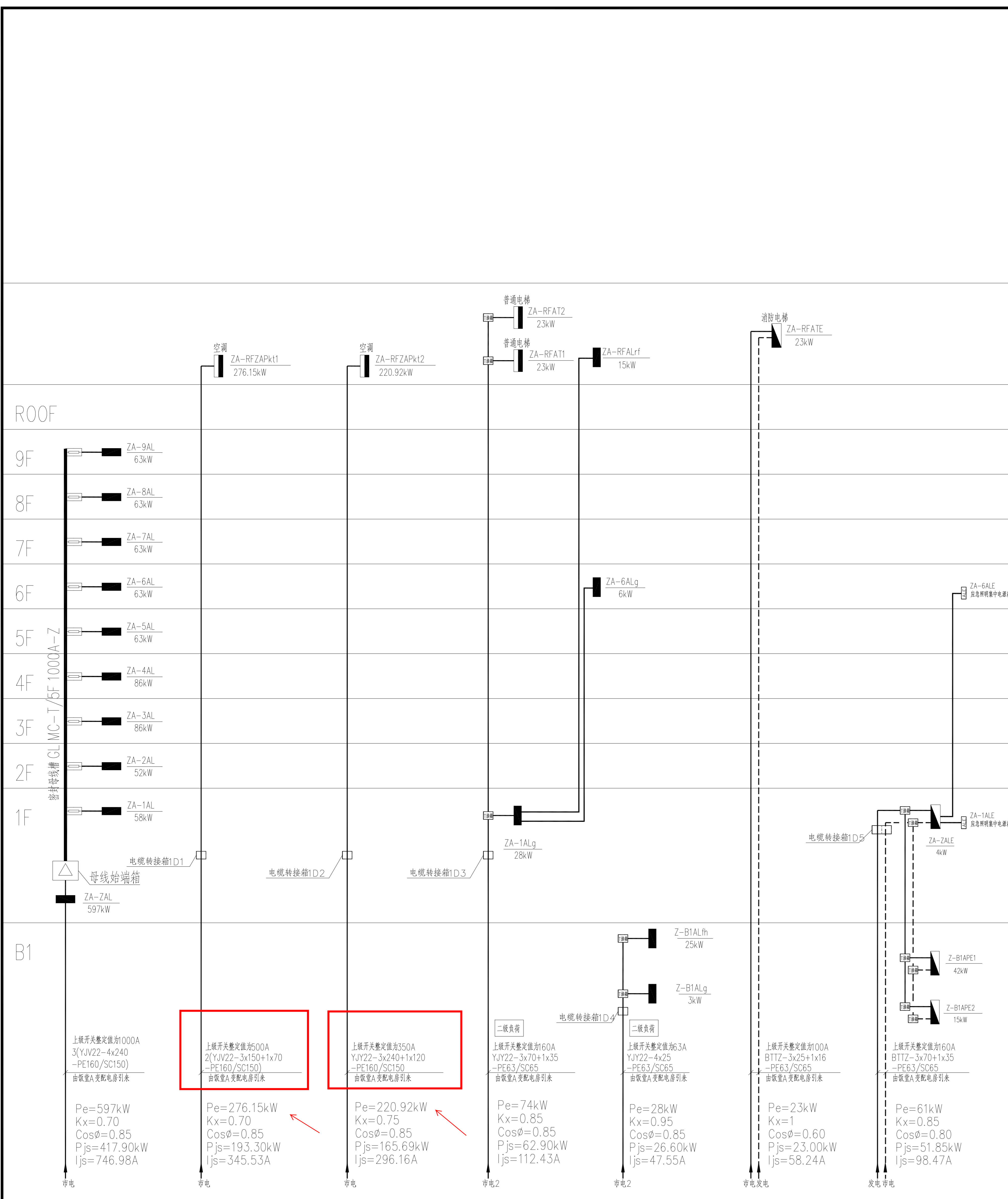
综合楼B A区电气竖向系统图
