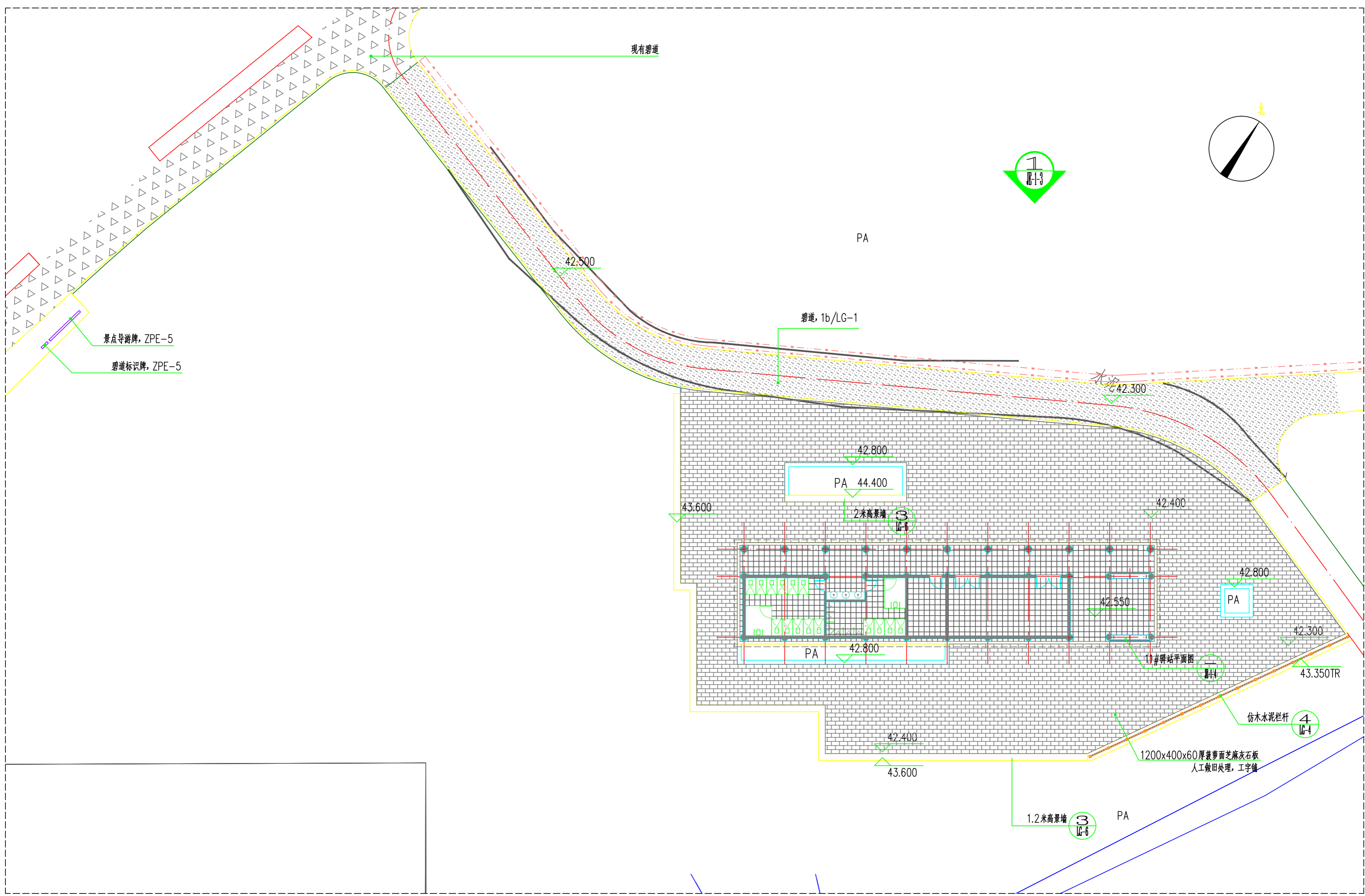
驿站三索引、铺装及标高平面图 1:200
