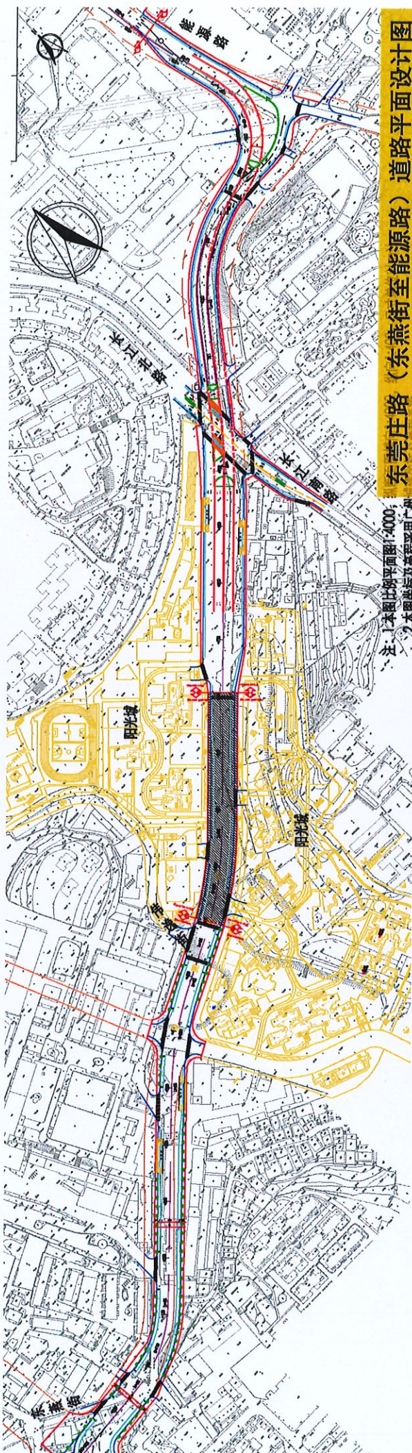
东莞庄路（广园路至东燕街）道路平面设计图
