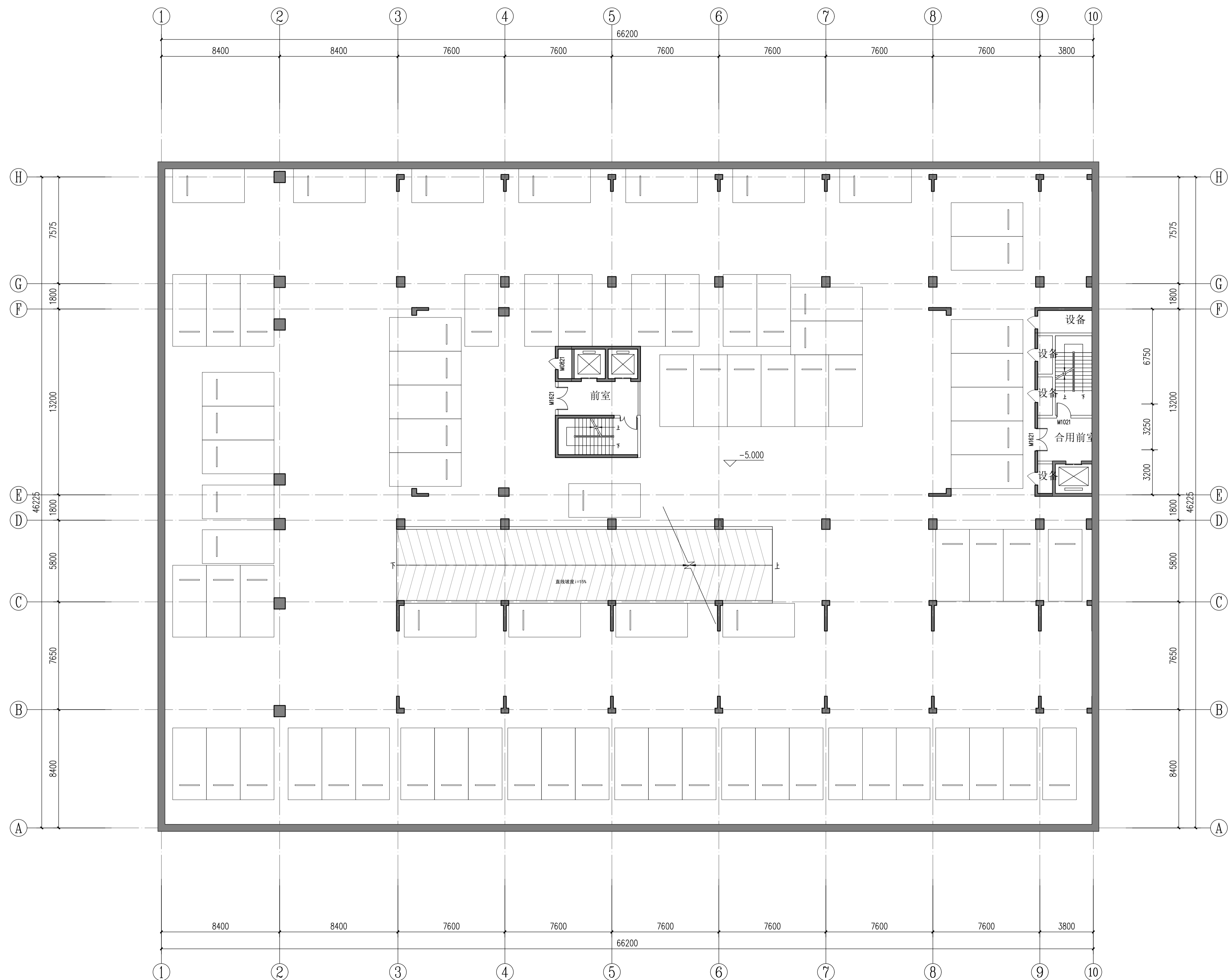
负一层(负150层)平面图
