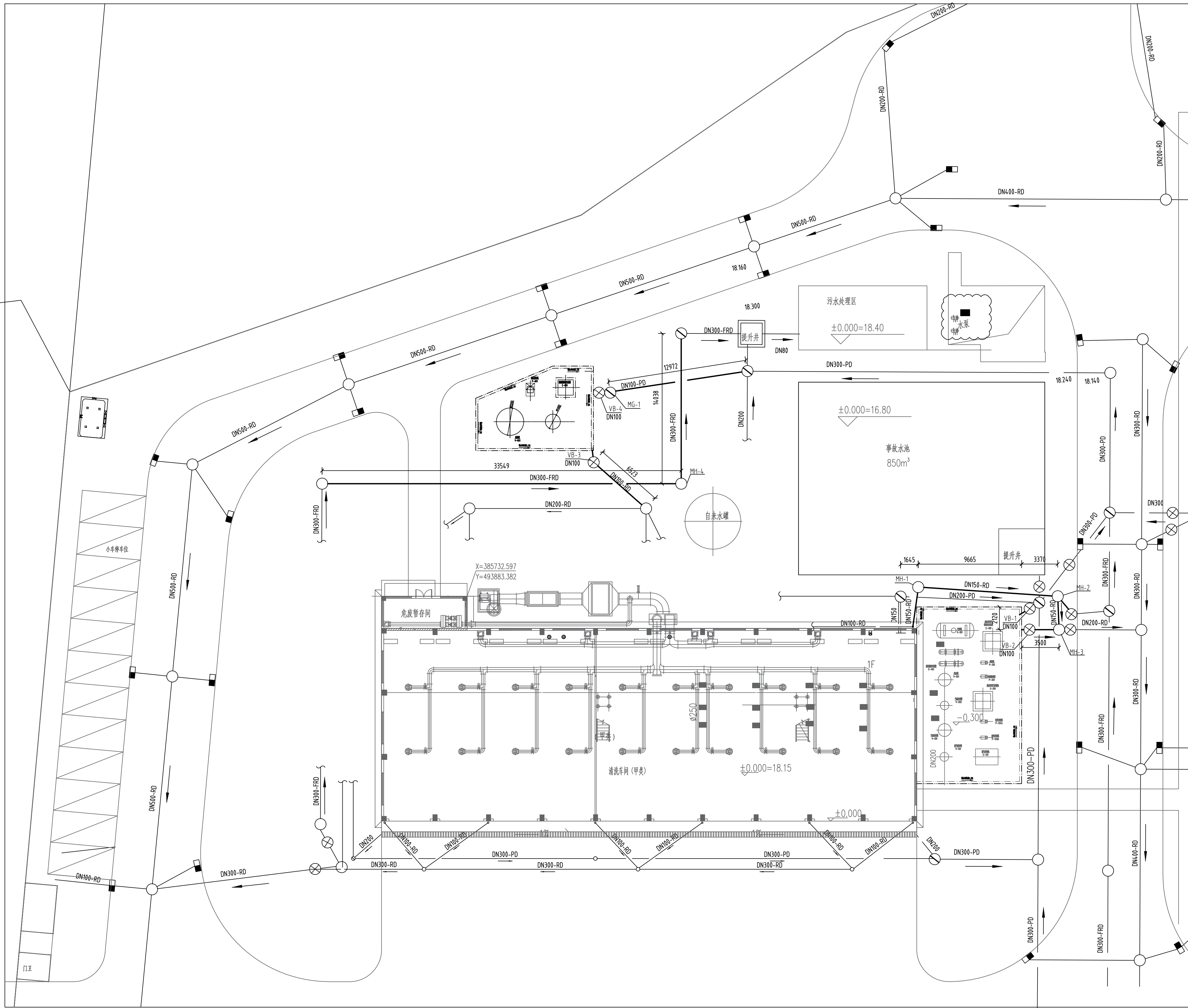
新增给排水管线平面布置图
